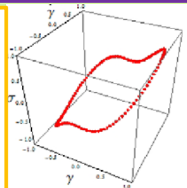
非線形領域におけるゴムのリサージュ曲線
